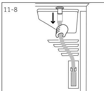
Tilkobling av avløpsslange
