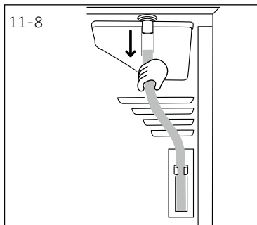
Anslutning av utloppsslangen
