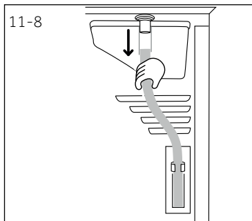
Tyhjennysletkun liitäntä
